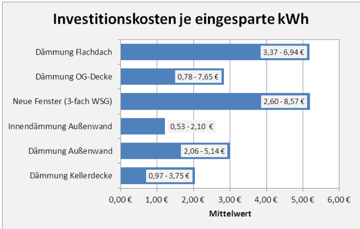
Abbildung 8: Investitionskosten je eingesparte Kilowattstunde Endenergie
