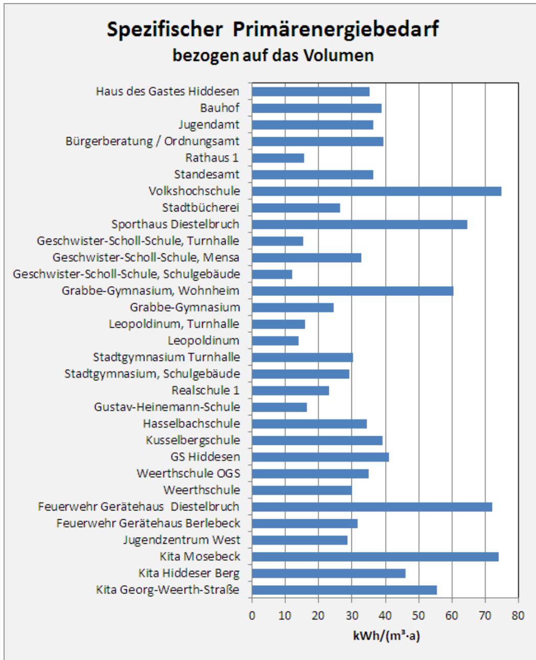
Abbildung 3: Spezifischer Primärenergiebedarf heute in kWh/(m³·a)
