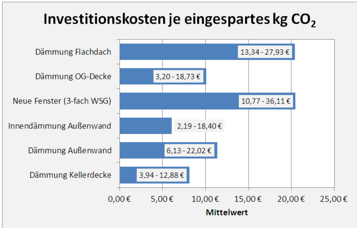
Abbildung 9: Investitionskosten je eingespartes Kilogramm CO 2
