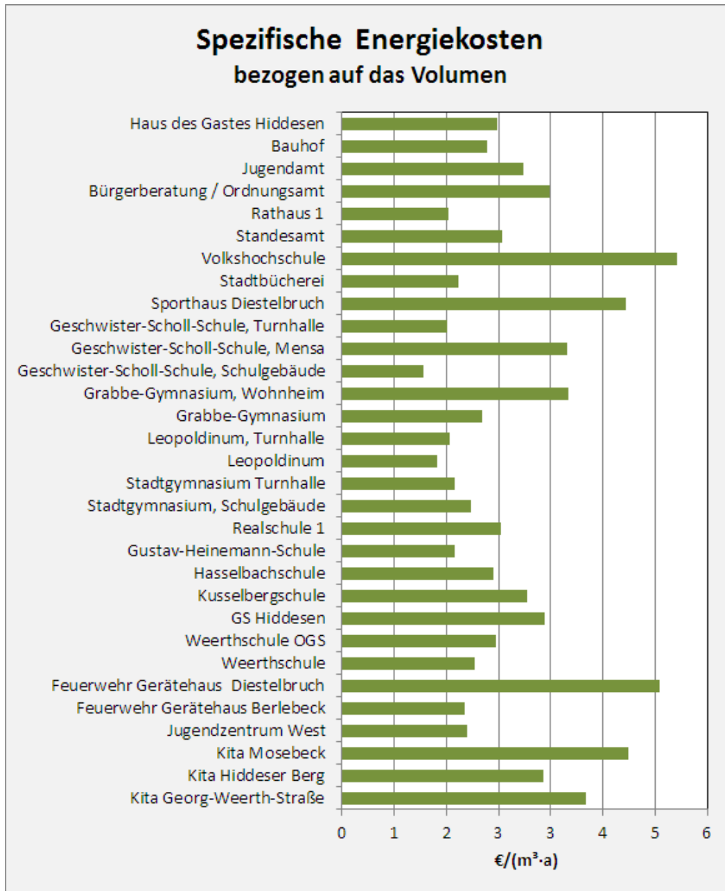
Abbildung 5: Spezifische Energiekosten heute in \text{€}/(\text{m}^3 \cdot \text{a})
